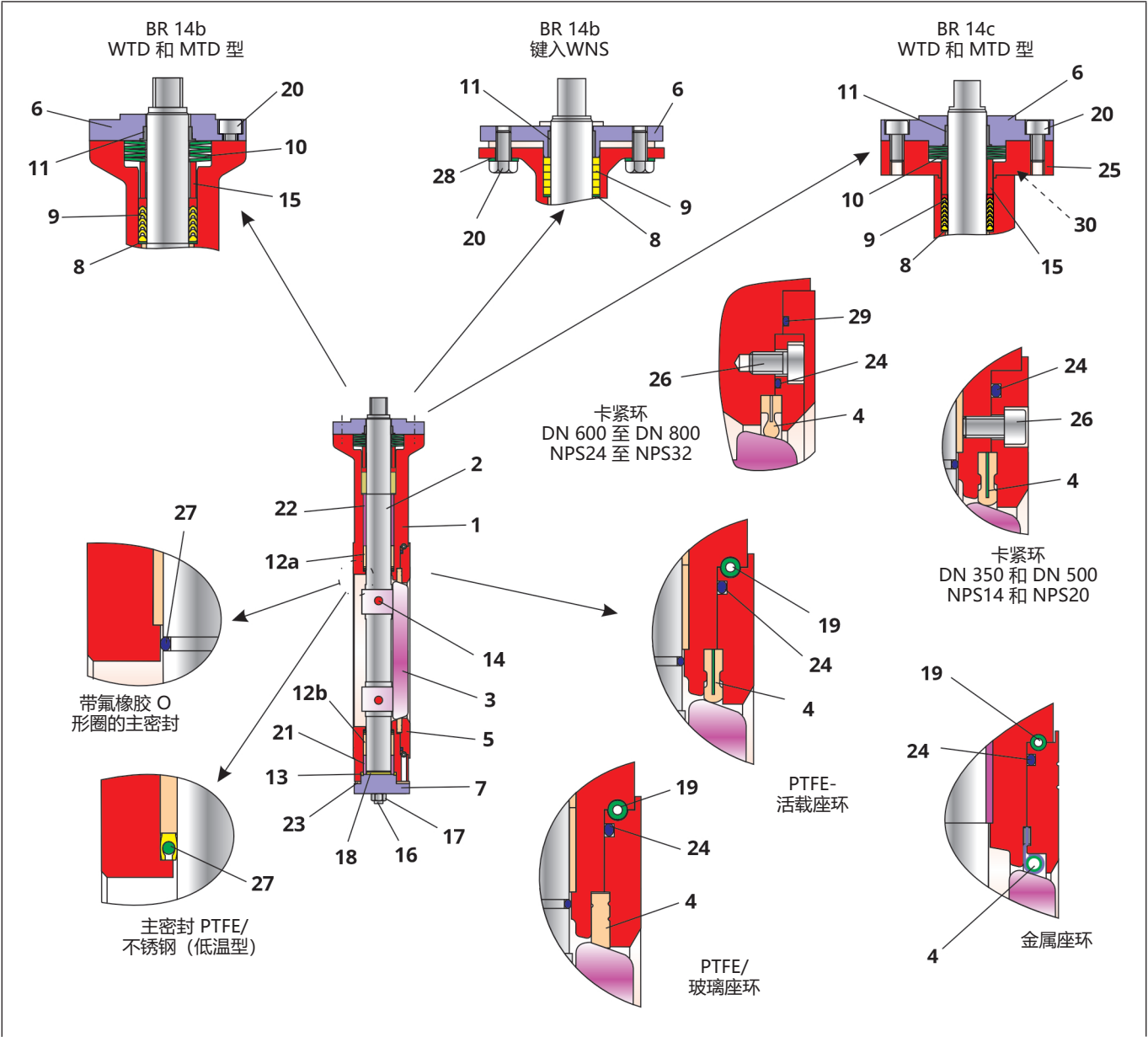
图 12-1: 蝶阀 BR 14b 剖面图
