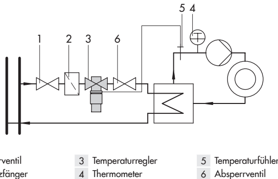
Bild 3-2: Einbaubeispiel Typ 43-6 an einem Kühler
