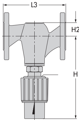
Flanschgehäuse (Sphäroguss)
