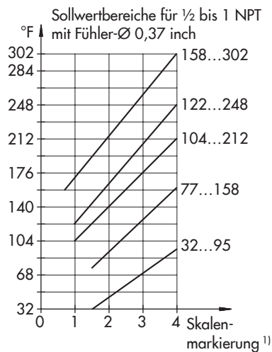
Typ 43-6 (ANSI)
