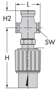
Innengewinde (Rotguss)
