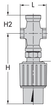
Innengewinde (Edelstahl)
