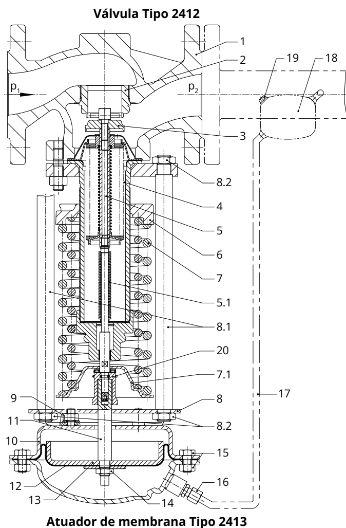
Fig. 4: Diagrama funcional para reguladores, DN 32 a 100 com fole de equilíbrio
