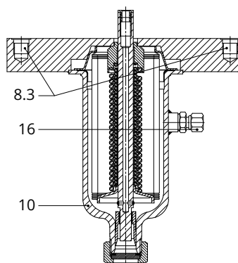
Atuador de fole ara DN 65 a 100
