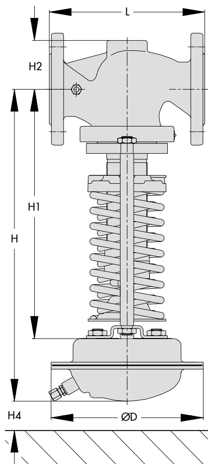
Tipo 41-23 com atuador de membrana
