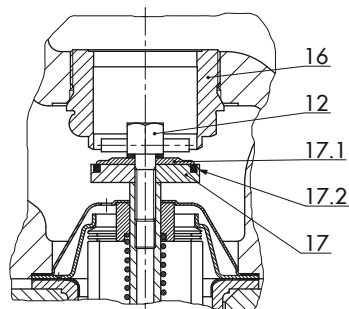
Versão com obturador com vedação macia
