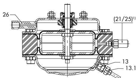
Fig. 6: Ligações do Tipo 2413 com atuador de membrana
