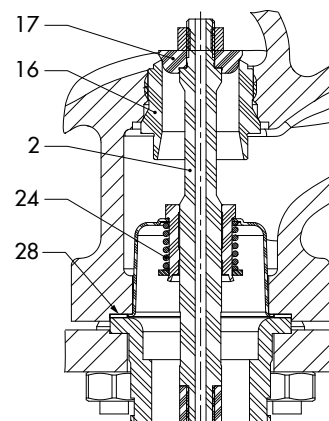
Standardausführung DN 15 bis 25
