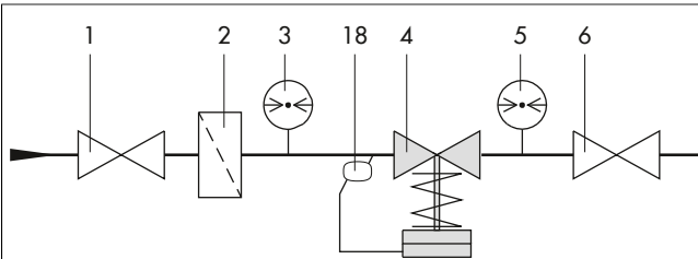
Bild 10: Universal-Überströmventil Typ 41-73, schematisches Einbaubeispiel
