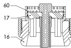
Ausführung mit Strömungsteiler
