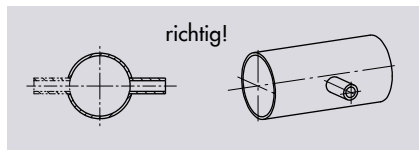
Bild 9: Steuerleitungsanschluss, abhängig von der Rohrführung
