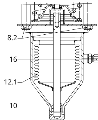
Balgantrieb für DN 15 bis 50
