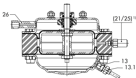
Bild 6: Anschlüsse Membranantrieb Typ 2413
