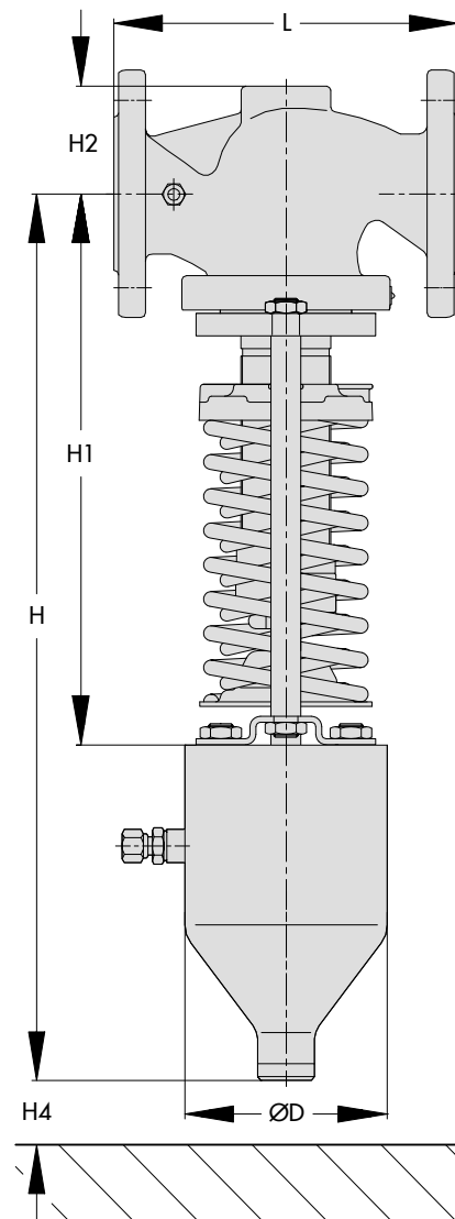
Typ 41-73 mit Balgantrieb
