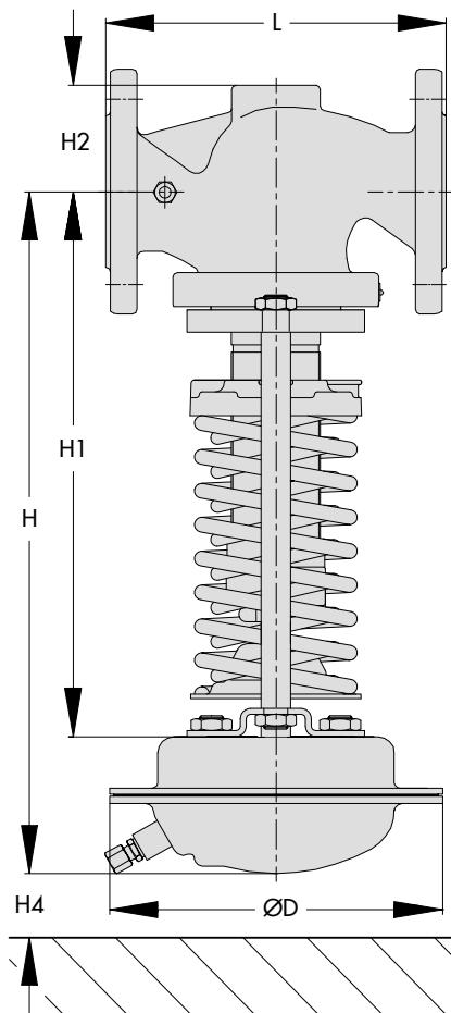
Typ 41-73 mit Membranantrieb
