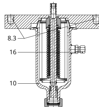
Balgantrieb Typ 2413
