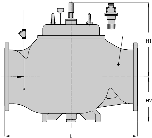
Ventil Typ 2422 · membranentlastet mit Pilotventil · DN 125 bis 400
