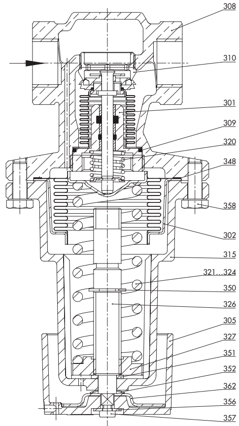
Rotgussgehäuse · Muffe
