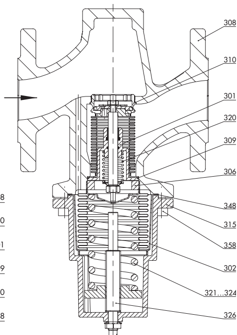
Sphärogussgehäuse · Flansch
