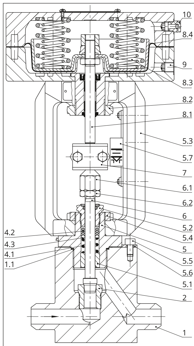
Bild 15: Schnittbild Typ 3252 mit eingeschraubtem Ventiloterteil und Antrieb Typ 3271 (120 cm 2 )
