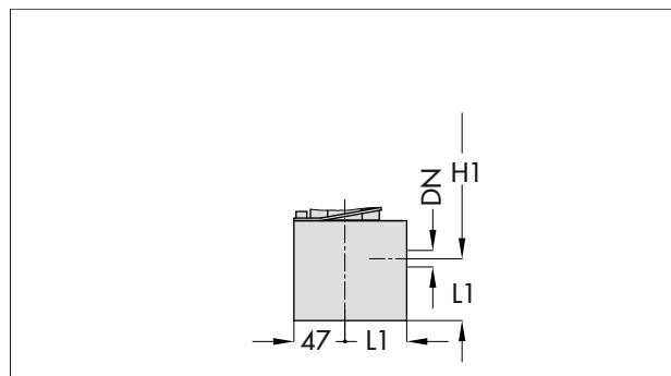
Bild 7: Eckventil Typ 3252 mit Innengewinde
