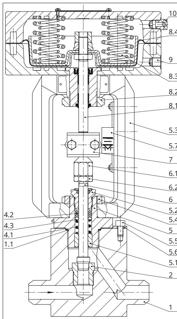
Bild 3: Schnittbild Typ 3252 mit eingeschraubtem Ventiloberteil und Antrieb Typ 3271 (120 cm 2 )
