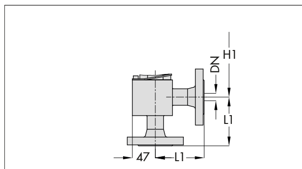
Bild 9: Eckventil Typ 3252 mit Flanschen
