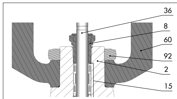
Bild 13: Packung mit Gewindebuchse zentral verschraubt (Beispieldarstellung)
