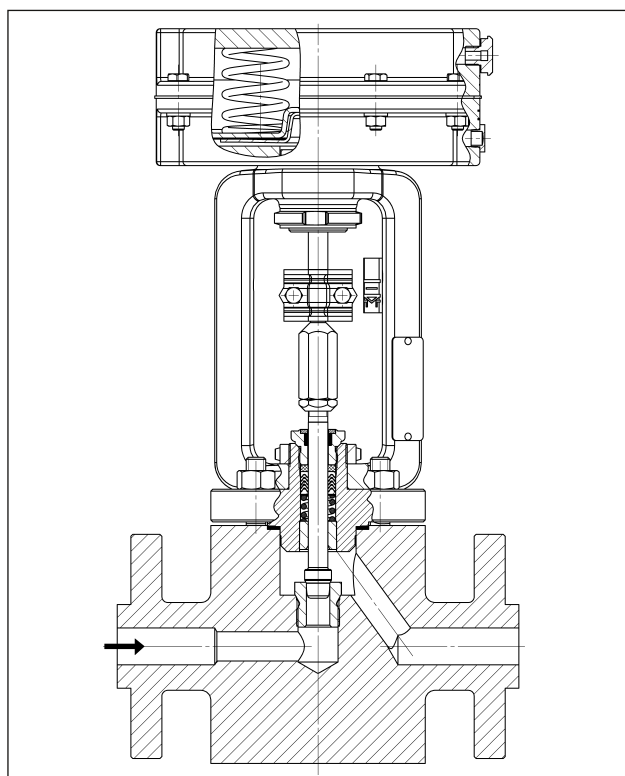
Bild 16: Schnittbild Typ 3252 mit angeflanschem Ventiloterteil und Antrieb Typ 3271 (120 cm 2 )
