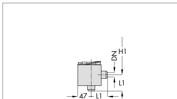
Bild 8: Eckventil Typ 3252 mit Anschweißenden
