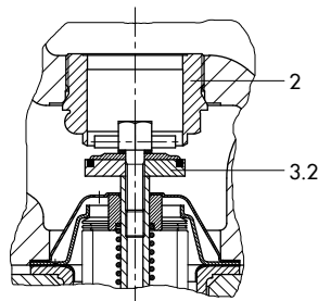
带软密封的阀芯
