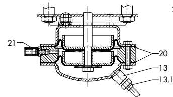
带两个安全增强型 膜片的膜片执行机构
