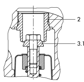
适用于小流量的阀门 K_{VS} \leq 2.5 : 不带平衡波纹管
