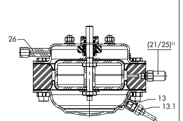
带两个高压灭菌器调节阀 膜片的膜片执行机构 (膜 片执行机构接头概览)
