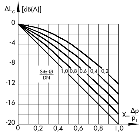
Bild 3: Diagramm · \Delta L_G bei Gasen und Dämpfen
