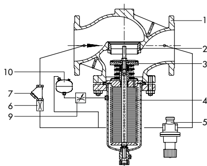
Druckminderer Typ 2333 (NPS 6 bis 10), Ventil Typ 2422 balgentlastet · Ausführung mit Ausgleichsgefäß und Nadeldrosselventil für Dampf (Nennweite DN 65 bis 100)
