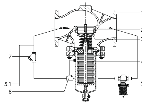
Überströmventil Typ 2335 (NPS 6 bis 10), Ventil Typ 2422 balgentlastet · Ausführung für flüssige und gasförmige Medien
