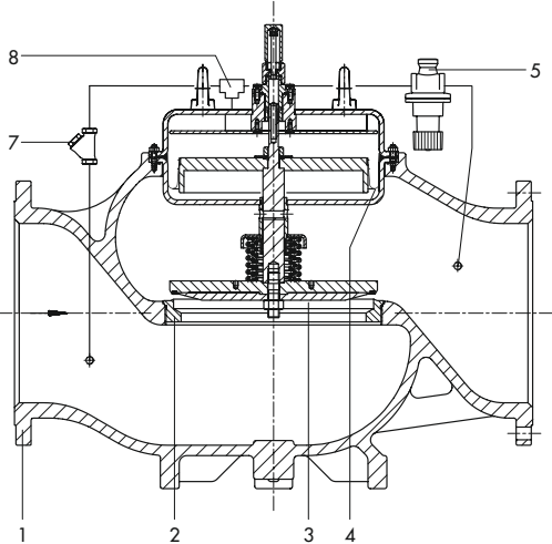
Druckminderer Typ 2333 (NPS 6, 8 und 10), Ventil Typ 2422 membranentlastet · Ausführung für flüssige und gasförmige Medien
