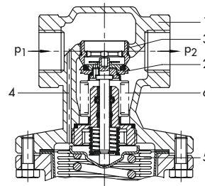
Überströmventil Typ 44-6 B · Muffengehäuse mit Innengewinde
