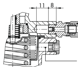
Edelstahl-/Sphärogussausführung (nur DN 40/50) und Sollwertbereich 8 bis 20 bar · Sollwerteinstellung über Innensechskantschraube
