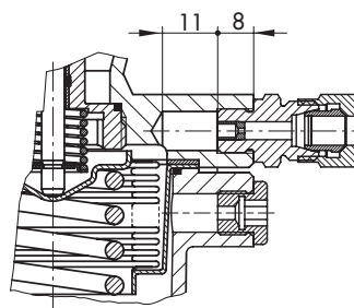
Sonderausführung Edelstahl Anschlussgewinde G \frac{1}{8} A für ein Manometer oder externe Steuerleitung · Maße in mm
