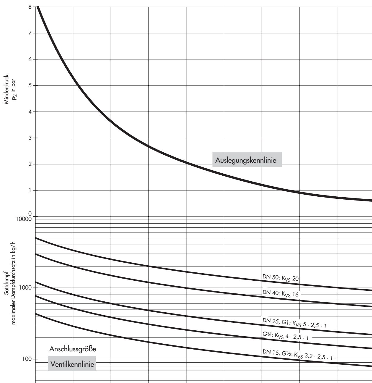
Bild 7: Diagramm zur Auslegung nach der Strömungsgeschwindigkeit
