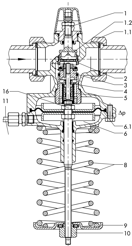
Bild 4: Typ 46-6 · Differenzdruck-Sollwert einstellbar von 0,2 bis 4 bar
