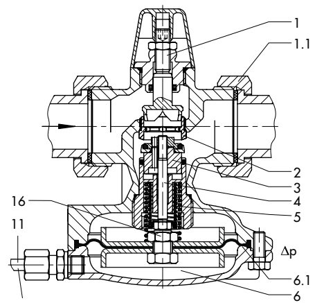
Bild 3: Typ 46-5 · Differenzdruck-Sollwert fest eingestellt
