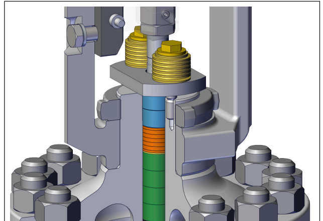
Bild 4: Packungsbrille selbstnachstellend (federbelastet außen) mit Nachziehooption
